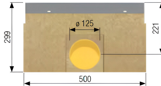
Poço de Inspeção em betão polímero
