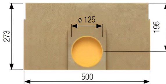
Poço de Inspeção em betão polímero
