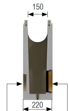
Secção "knock-out" para ponto adicional de drenagem \varnothing 160 Manga com vedação \varnothing 160
